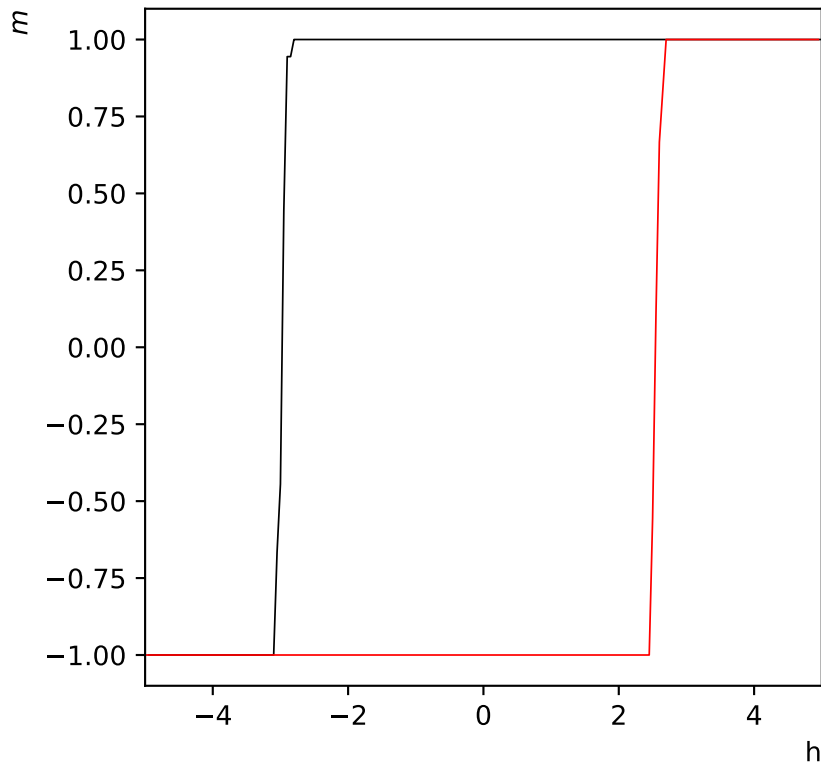
Hystérésis de l'aimantation réseau de taille L=6 - h=5 à T=0.5
