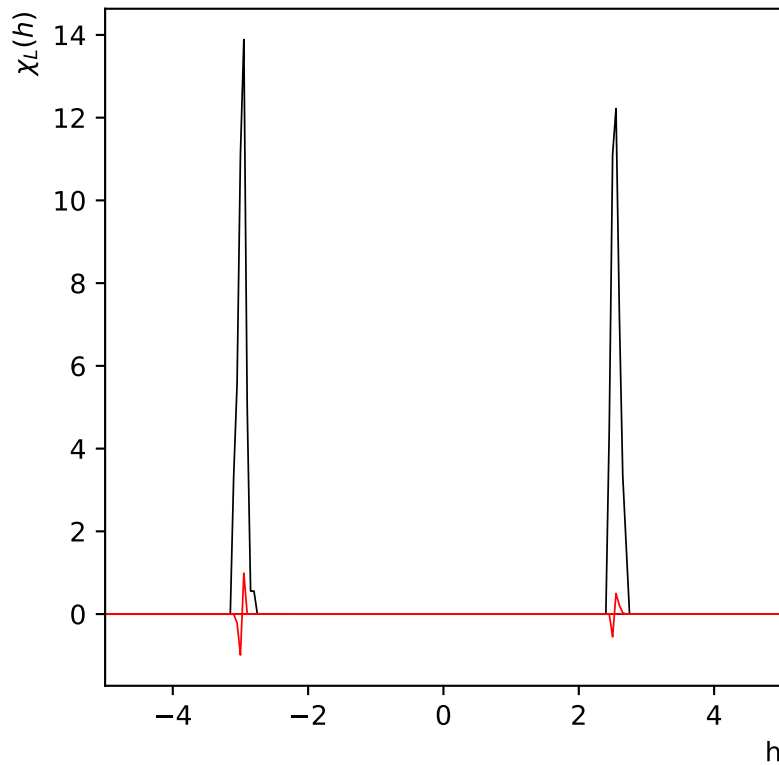
\chi_L(h) réseau de taille L=6 à T=0.5
